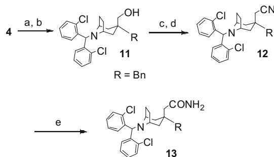
Scheme 4. Reagents and conditions: (a) DIBAL in toluene, 0^\circ\text{C} ; (b) \text{NaBH}_4 , MeOH, 0^\circ\text{C} ; (c) \text{MsCl} , \text{Et}_3\text{N} , DCM, 0^\circ\text{C} ; (d) \text{KCN} , 18-crown-6, DMF, 110^\circ\text{C} ; (e) concd \text{H}_2\text{SO}_4 , neat, rt.
